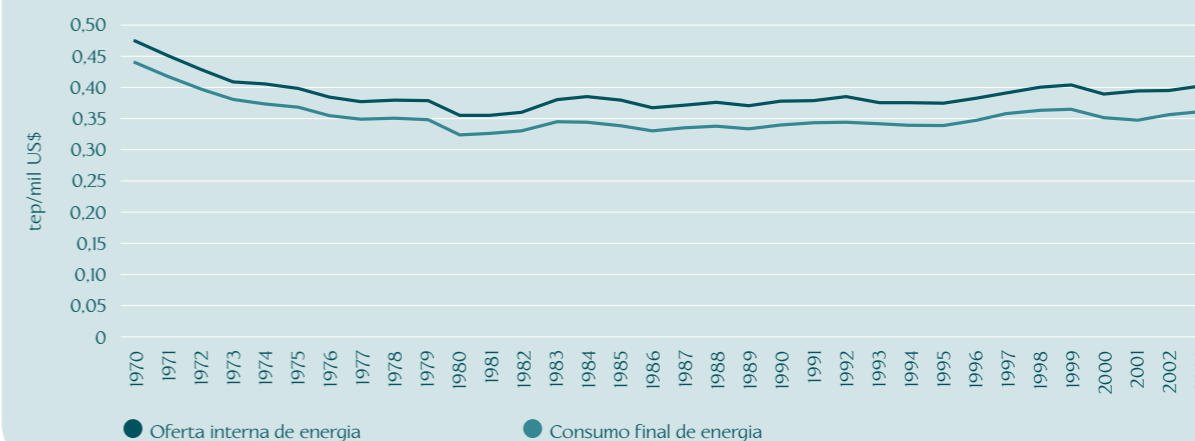
GRÁFICO 4 • Medidas de intensidade no uso de energia, calculadas a partir de dados de oferta de energia e consumo de energia – Brasil, 1970 a 2003
