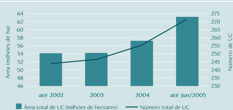
GRÁFICO 2 • Número e área total de Unidades de Conservação federais – Brasil, 2002 a 2005
