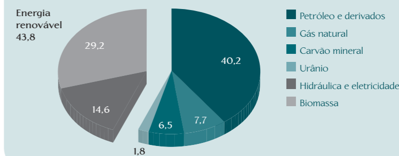
GRÁFICO 5 • Participação relativa das fontes na oferta interna de energia – Brasil, 2003 (em %)
