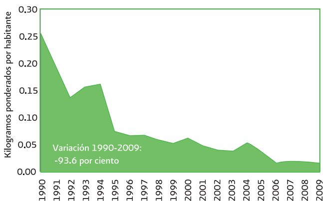
GRÁFICA 7.3. CONSUMO DE SUSTANCIAS QUE AGOTAN LA CAPA DE OZONO, 1990 A 2009
