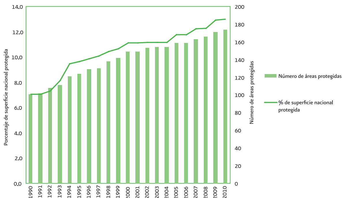
GRÁFICA 7.5. ÁREAS TERRESTRES Y MARINAS PROTEGIDAS, 1990 A 2010
