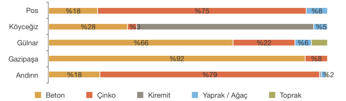
Grafik 25. Bölgelere Göre Çatı Malzemesi
