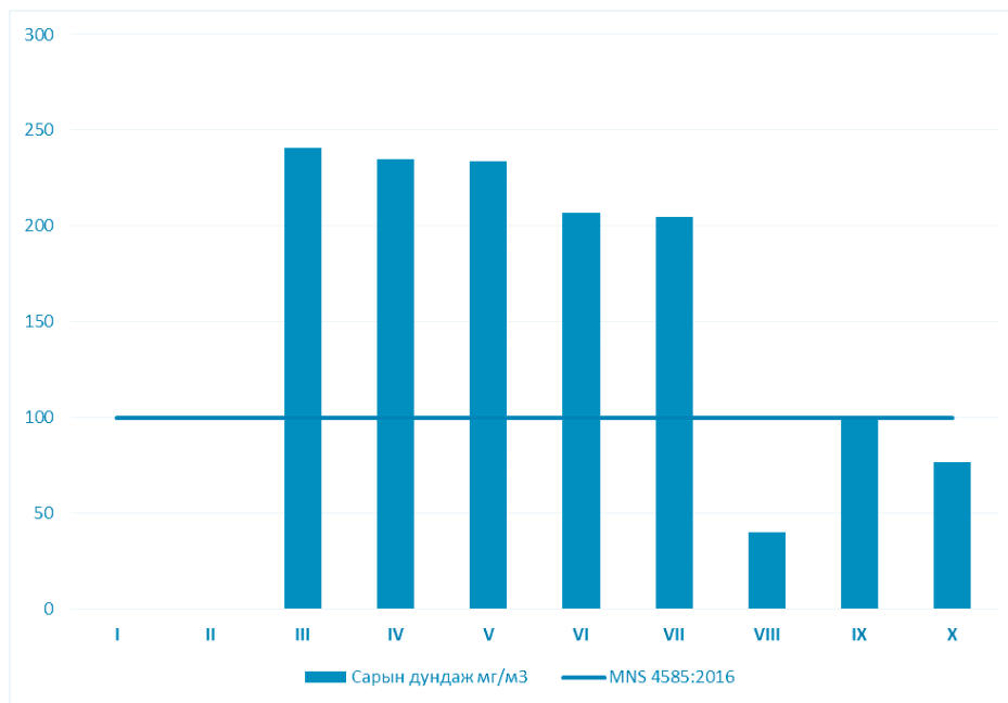
Дүрслэл 11. Цогтцэций сумын цаг уурын ажиглалтын харуулаас сумын төв орчмын агаар дахь PM10 буюу том ширхэгт тоосонцорыг хэмжсэн дүн, 2017 он
