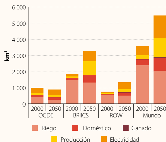
Demande mondiale en eau (prélèvements d'eau douce) : scénario de base, 2000 et 2050
