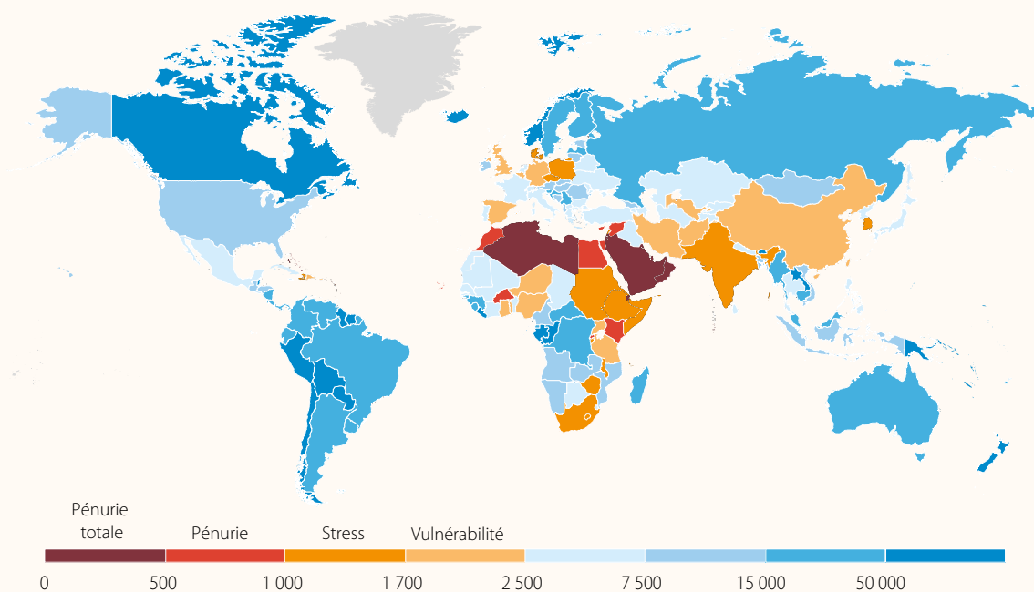
Total des ressources en eau renouvelables, 2011 (m 3 par habitant et par année)
