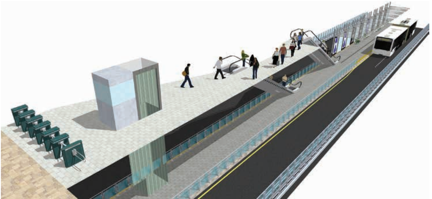
Рисунок 70 Проектное решение, направленное на увеличение пропускной способности и сокращение переполненности остановочного комплекса, размещенного на центральной разделительной полосе в системе БРТ, организованной на скоростной автомагистрали (обратите внимание, что это концептуальный набросок организации пассажирского доступа, и на нем не отображены все рекомендуемые ограждающие конструкции).
