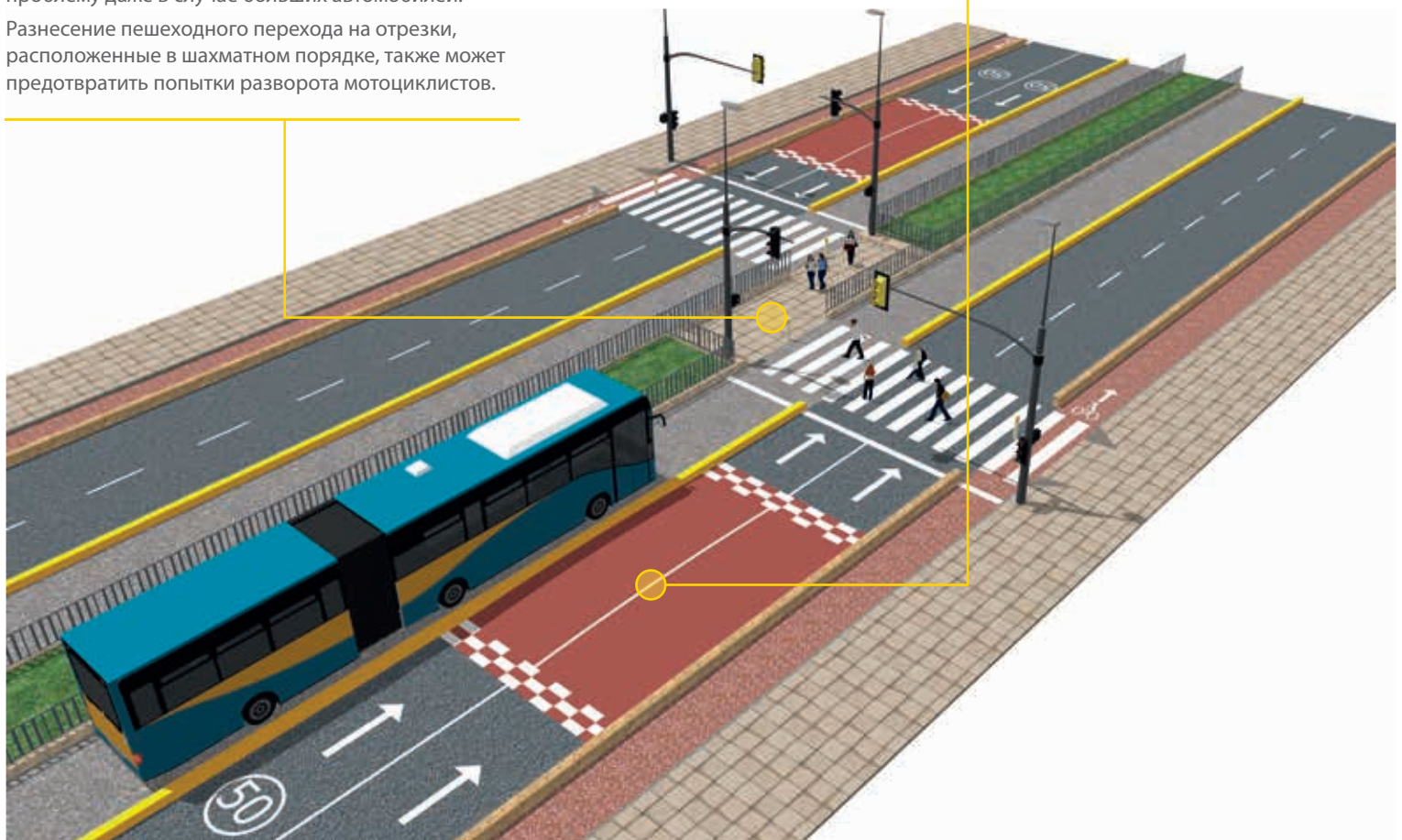
Рисунок 9 Пешеходный переход на перегонном участке городской магистрали
