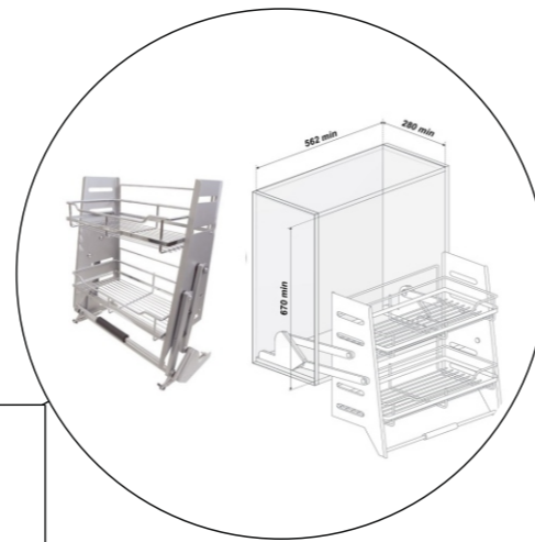
Лифтовая корзина
