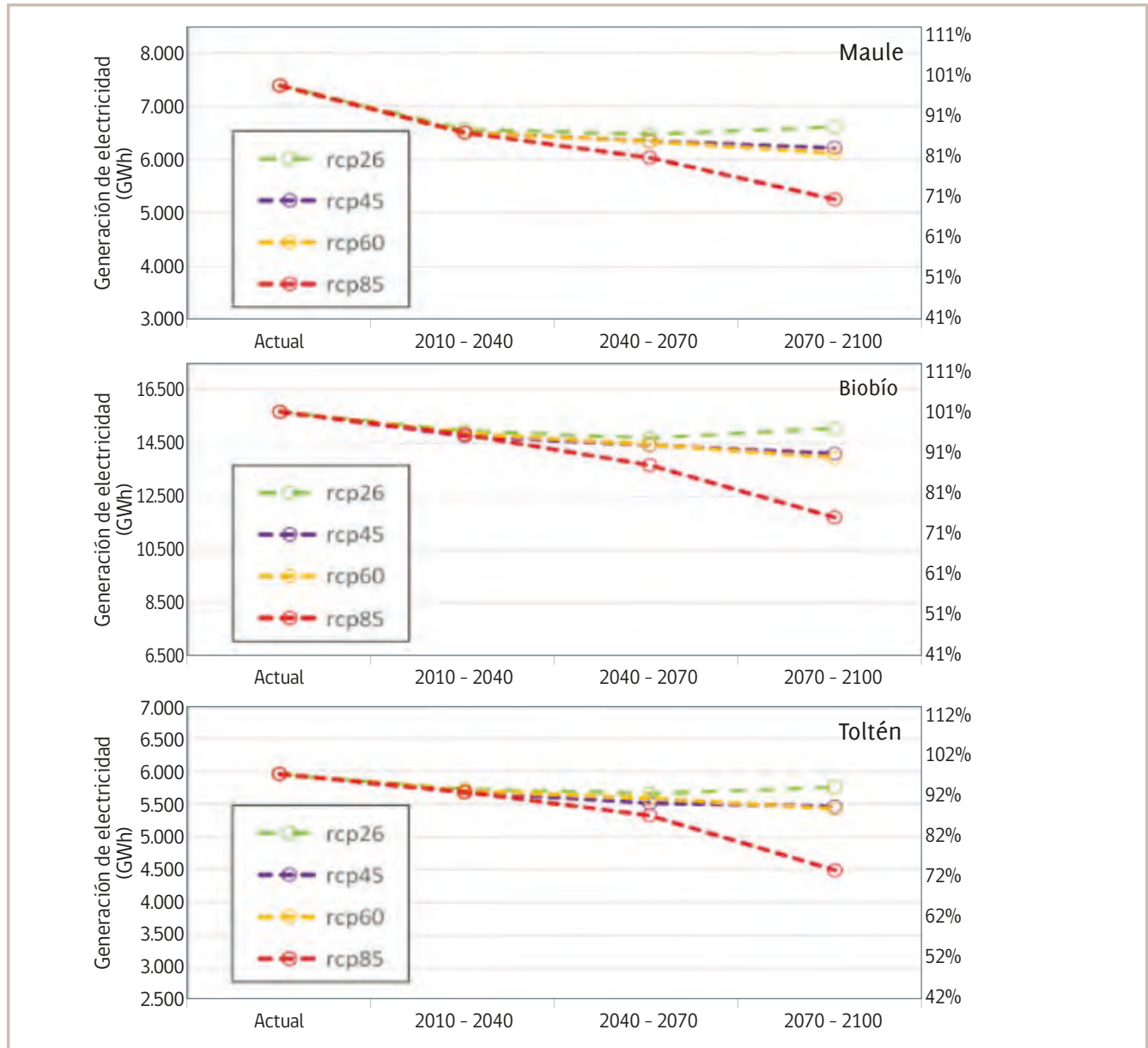
Figura 11. Estimación del impacto del cambio climático en la capacidad de generación de electricidad asociada a proyectos futuros en las cuencas de Maule, Biobío y Toltén
