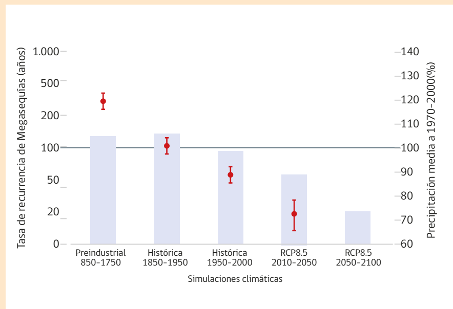
Figura 3-7. Período de recurrencia en años (escala a la izquierda) de una sequía (> 30% de déficit de precipitación en Chile central) de tres o más años de duración, empleando siete modelos climáticos que simulan climas pasados, presentes y futuros. El período de recurrencia se calculó para cada modelo. Los círculos rojos indican el promedio y las líneas verticales la desviación estándar entre modelos. Las barras celestes indican el promedio multimodelo de la precipitación relativa a la media 1970-2000 (escala a la derecha)
