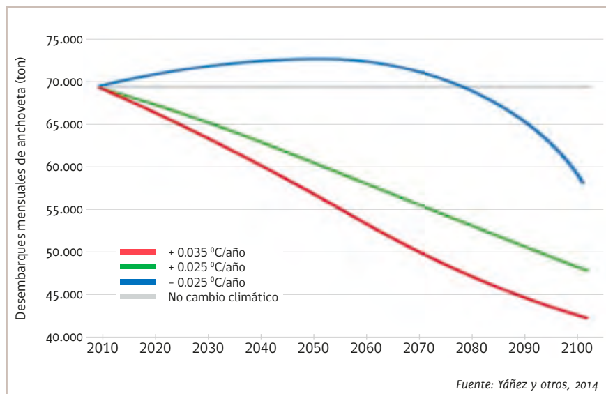
Figura 3-20. Proyección mensual de los desembarques de anchoveta en la zona norte de Chile, considerando cuatro escenarios de cambio climático.
