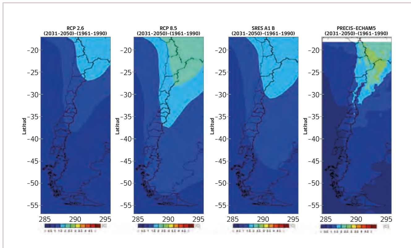
Figura 3-4. Mapas de cambio de temperatura para escenarios RCP y SRES A1B (GCM y RCM) para el período 2031-2050 en comparación con el período 1961-1990
