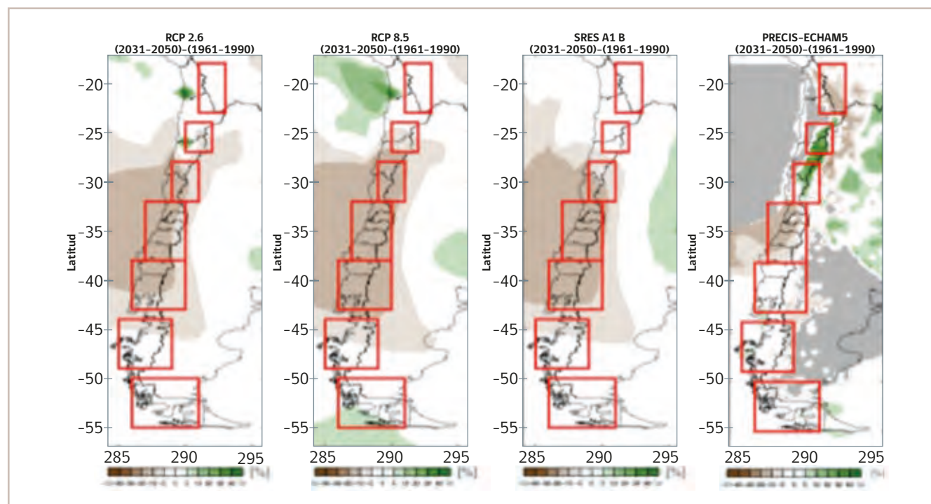
Figura 3-5. Mapas de cambio de precipitaciones para escenarios RCP y SRES A1B (GCM y RCM) para el período 2031-2050 en comparación con el período 1961-1990
