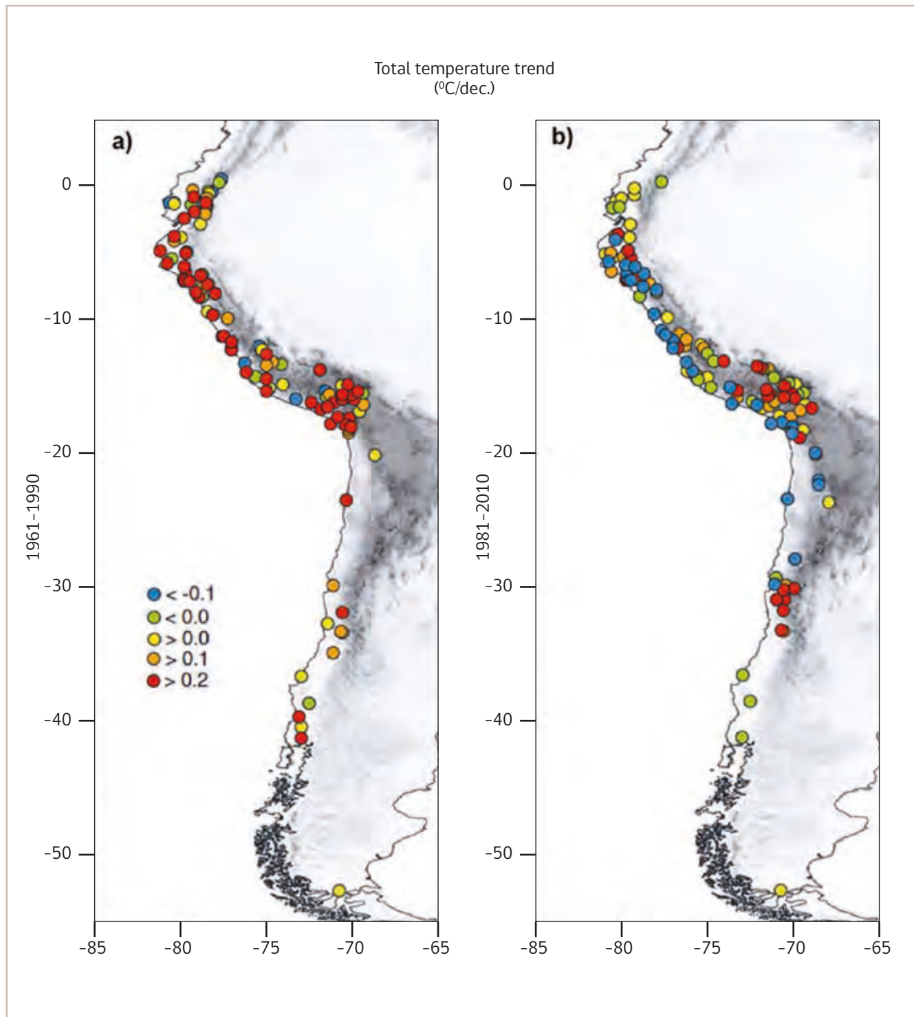
Figura 3-1. Análisis de tendencia en temperatura.
